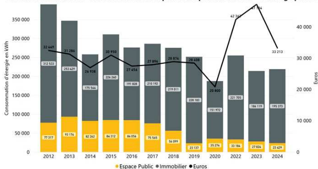
Evolution annuelle des consommations et dépenses du patrimoine bâti + éclairage public
